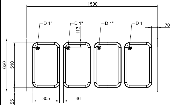
Boven aanzicht
