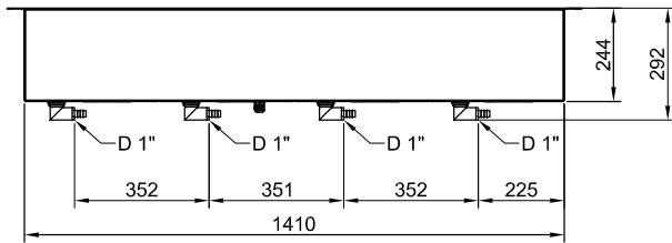
Zij aanzicht
